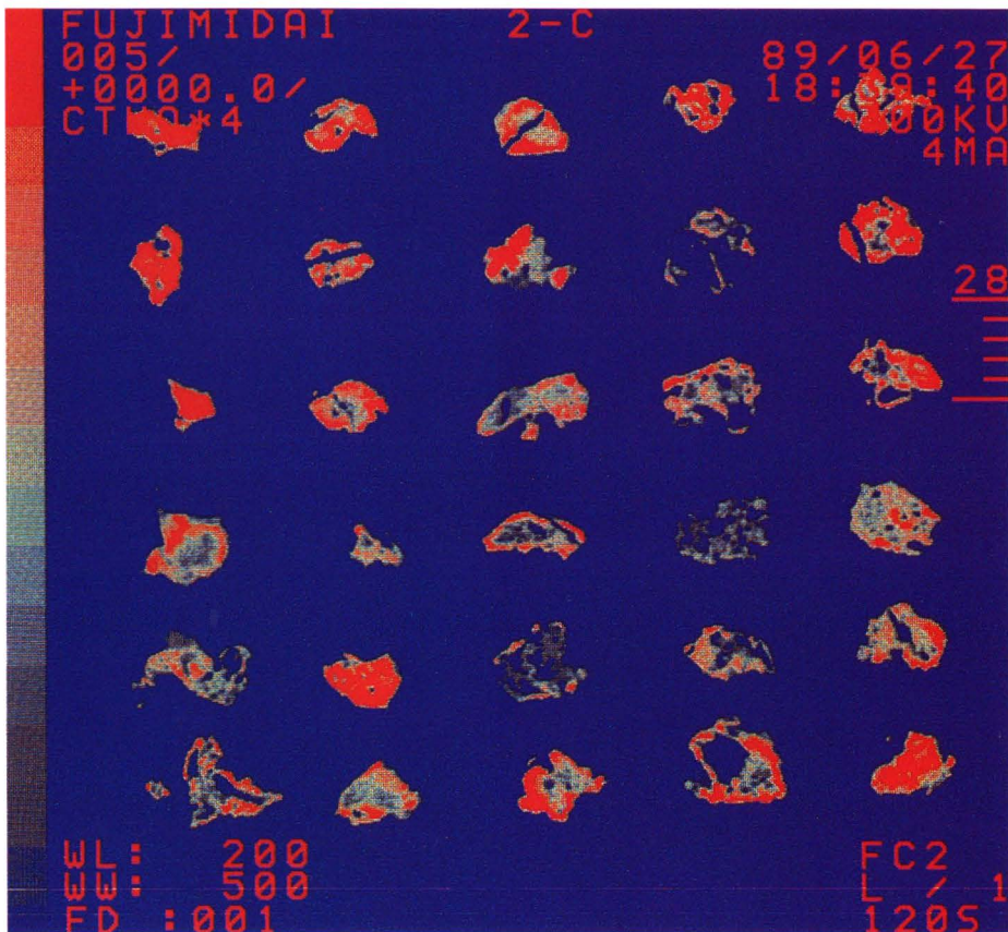
千葉県富士見台第II遺跡C地点出土鉄塊系遺物写真とX線CT写真
