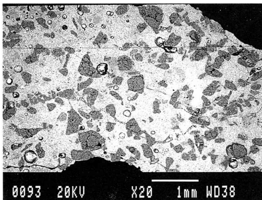
蓮代寺3-1 (S93A) マクロ組織
