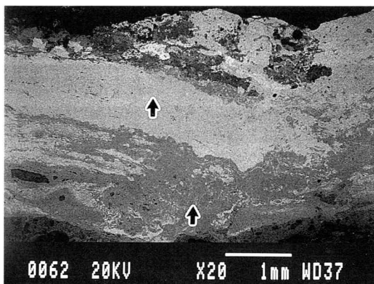
北栗2 (T62C) マクロ組織
