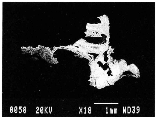
玉田8号墳2 (T58B③) マクロ組織
