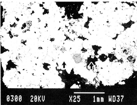
板井砂奥1 (S300) マクロ組織
