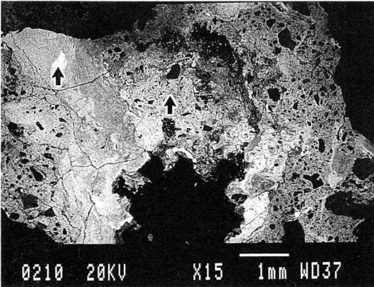
脇田6 (S210) マクロ組織
