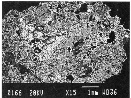
丹摩古墳3 (S166) マクロ組織
