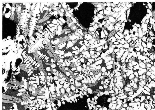
勝山館14 (S129) ミクロ組織 a 2
