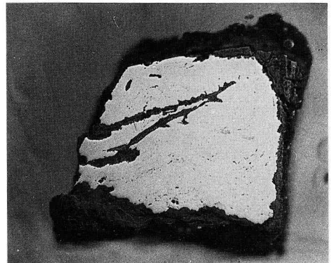
勝山館23B (T68) マクロ組織
