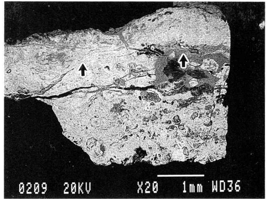
脇田6 (S209) マクロ組織
