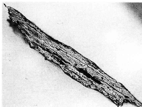
勝山館21 (T66) マクロ組織
