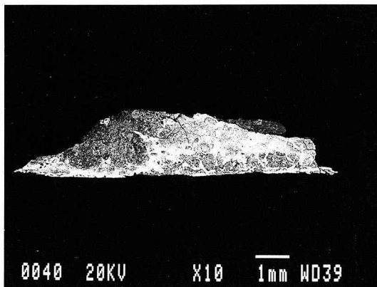
金海七山洞古墳1 (T40B③) マクロ組織
