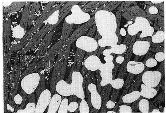
勝山館6 (S113) ミクロ組織 a 2
