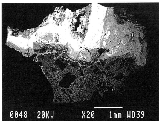
蔚山下袋1 (T48A③) マクロ組織
