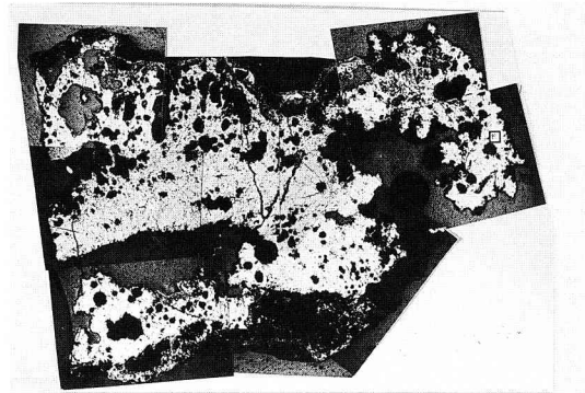
勝山館6 (S113) マクロ組織
