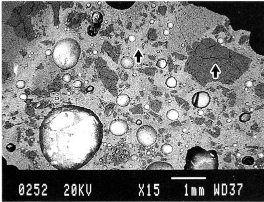
大県84-1-3 (S252) マクロ組織
