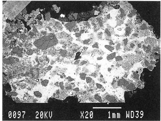
蓮代寺3-8 (S97A) マクロ組織
